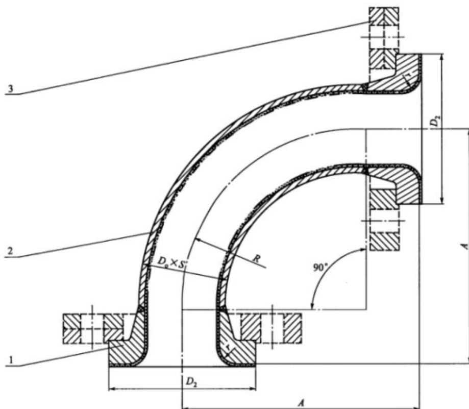
图 1 搪玻璃 90°弯头结构型式图
